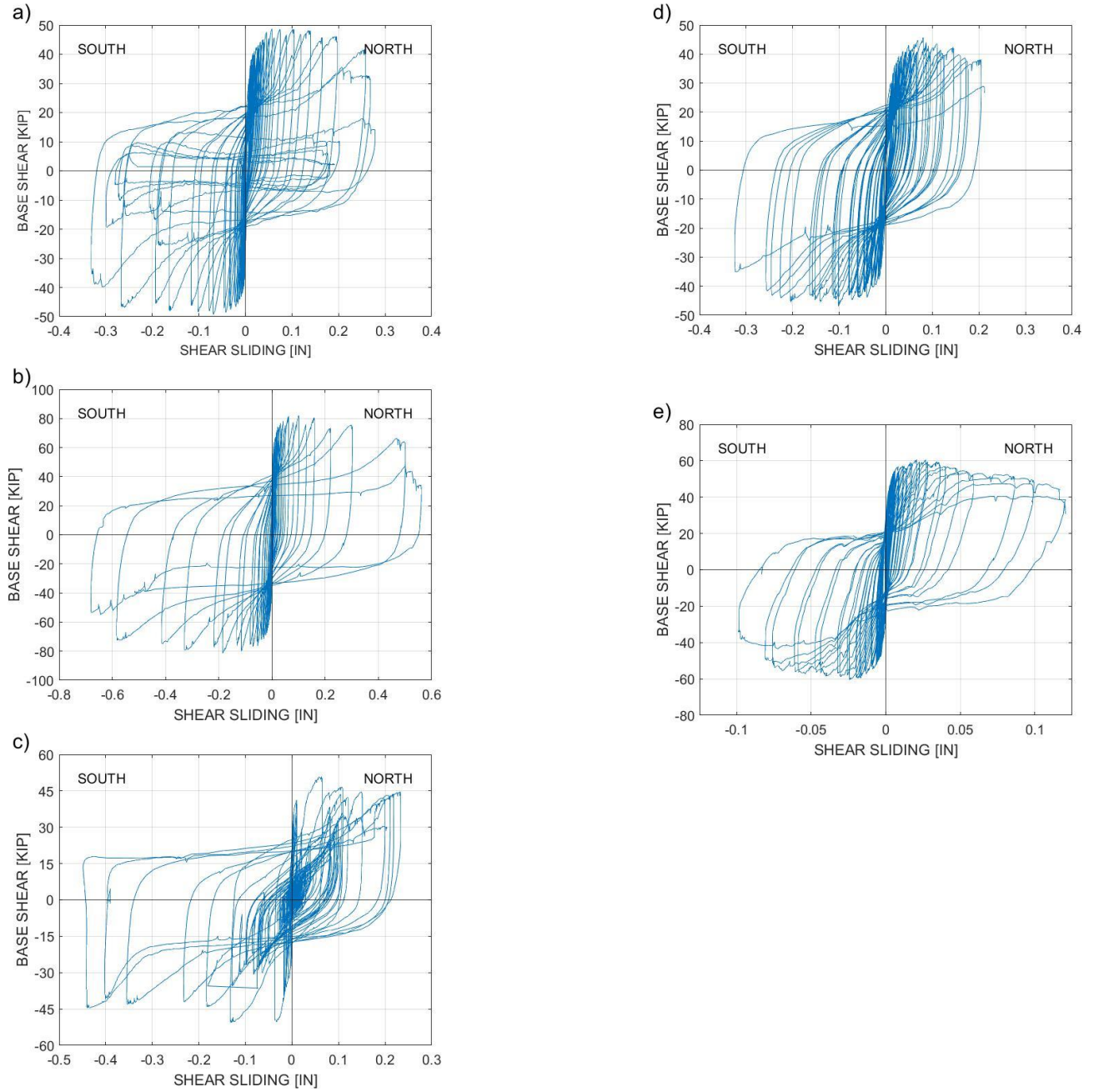
Figure 3.44. Shear Sliding: a) C(CFRP)-4.0-#5(1.4)-0.05, b) C(CFRP)-4.0-#7(2.7)-0.05, c) C(CFRP)-4.0-#7(1.3)-0.05-EQ, d) C(CFRP)-4.0-#7(1.3)-0.05-2X, e) C(CFRP)-4.0-#7(1.3)-0.15
