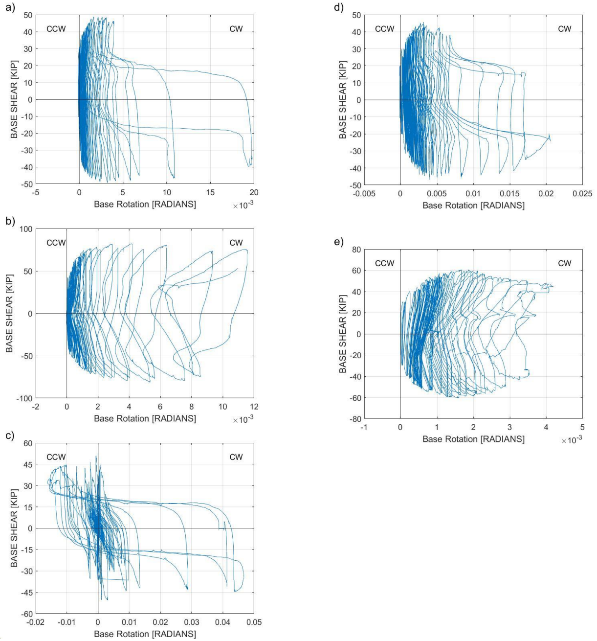
Figure 3.45. Base Rotation: a) C(CFRP)-4.0-#5(1.4)-0.05, b) C(CFRP)-4.0-#7(2.7)-0.05, c) C(CFRP)-4.0-#7(1.3)-0.05-EQ, d) C(CFRP)-4.0-#7(1.3)-0.05-2X, e) C(CFRP)-4.0-#7(1.3)-0.15
