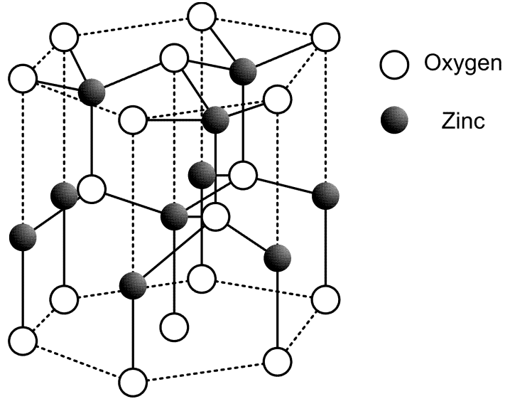
FIG. 1.1. Wurtzite ZnO.
