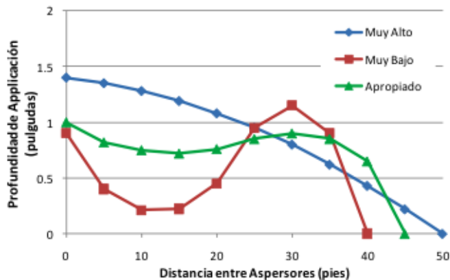
Figura 7. Profundidades de aplicación (patrones) con respecto a la distancia de un aspersor por presiones que van desde muy alta a muy baja y las que están ajustadas apropiadamente.
