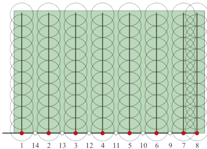
Figura 4. Mostrando la forma de movimiento de SKIP. Regar de cada tercer hidrante hacia abajo de la parcela (rojo), luego regar de regreso de los hidrantes que no se regaron (blanco) (Hidrantes 1-14 en orden)
