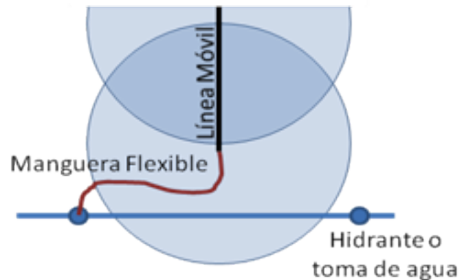
Figura 5. Utilizando una adaptación "fuera de sitio" en cada tercer ciclo de riego puede mejorar significativamente la uniformidad de aplicación.
